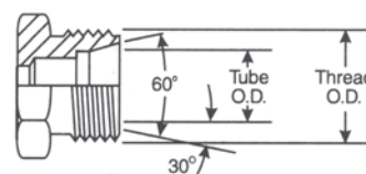
Male 60° Cone, DIN 7611
